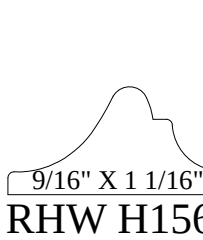
9/16" X 1 1/16" RHW H156
